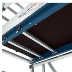
Plancher alu-bois à plinthes rapportées
